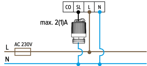
Kytcentä suoraan verkkovirtaan
