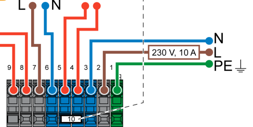
LAVI COOL -kytkennät
